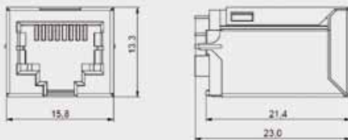
Y-ConJack-22-THR
