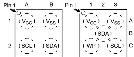
WLCSP-4**
