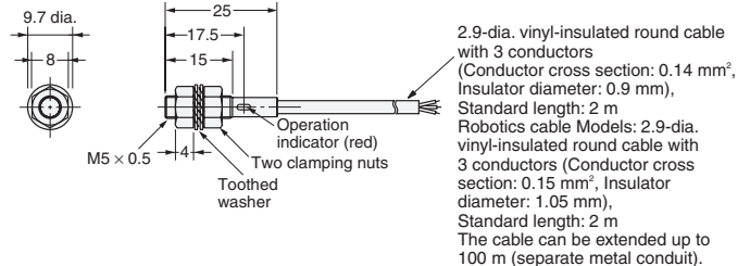
Fig. 4: E2E-X1□□
