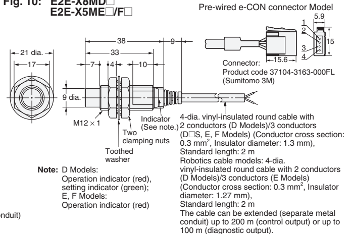
Fig. 10: E2E-X8MD□ E2E-X5ME□/F□
