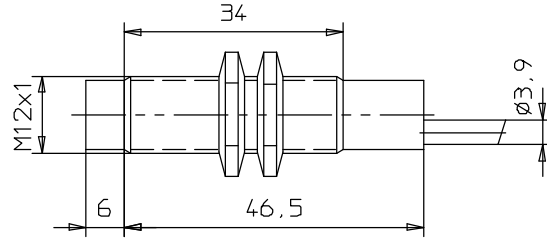
E2EL-X8M□
