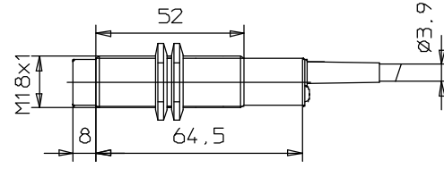
E2EL-X15M□
