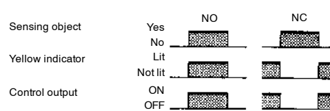
E2EL-X□F□ PNP Output
