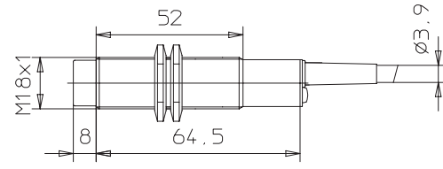
E2EL-X8M□-L 2M
