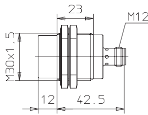
E2EL-X15M□-M1
