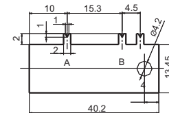
F29(h=1,R=500), F30(h=2,R=250)
