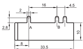
F39(h=1,R=700), F40(h=2,R=350)
