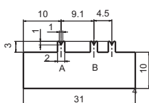
F33(h=1,R=400), F34(h=2,R=200)
