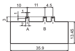
F25(h=1,R=380), F26(h=2,R=190)
