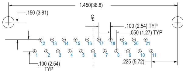
21 SOCKET M83513/19-C
