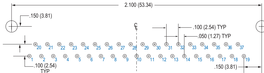
37 SOCKET M83513/19-F
