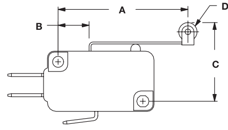
FIG. 2 Lever Roller
